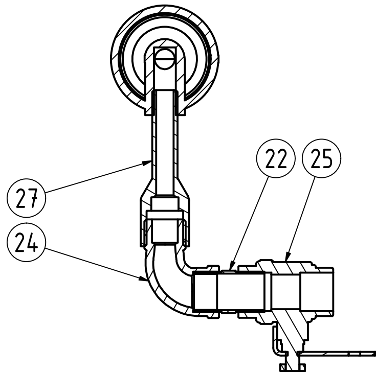
B-B ( 1 : 2 )
