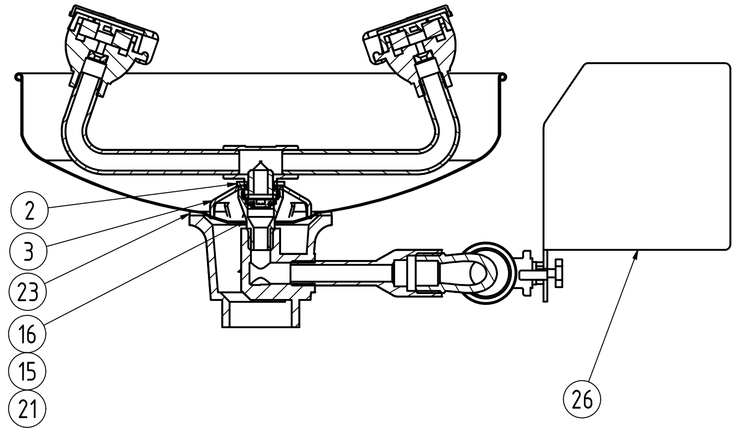
A-A ( 1 : 2 )
